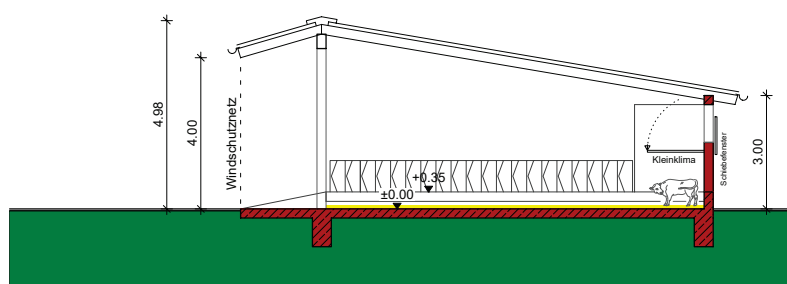
Längsschnitt
