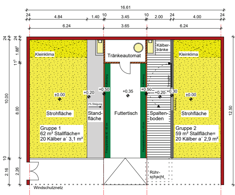
Grundriss Stallebene mit Standfläche oder Spaltenboden
