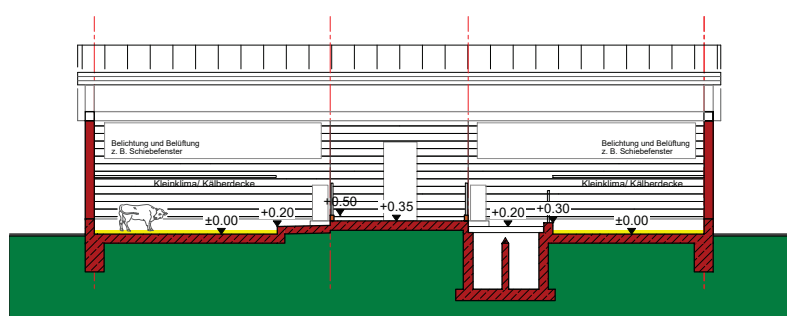
Querschnitt Bodenprofil
