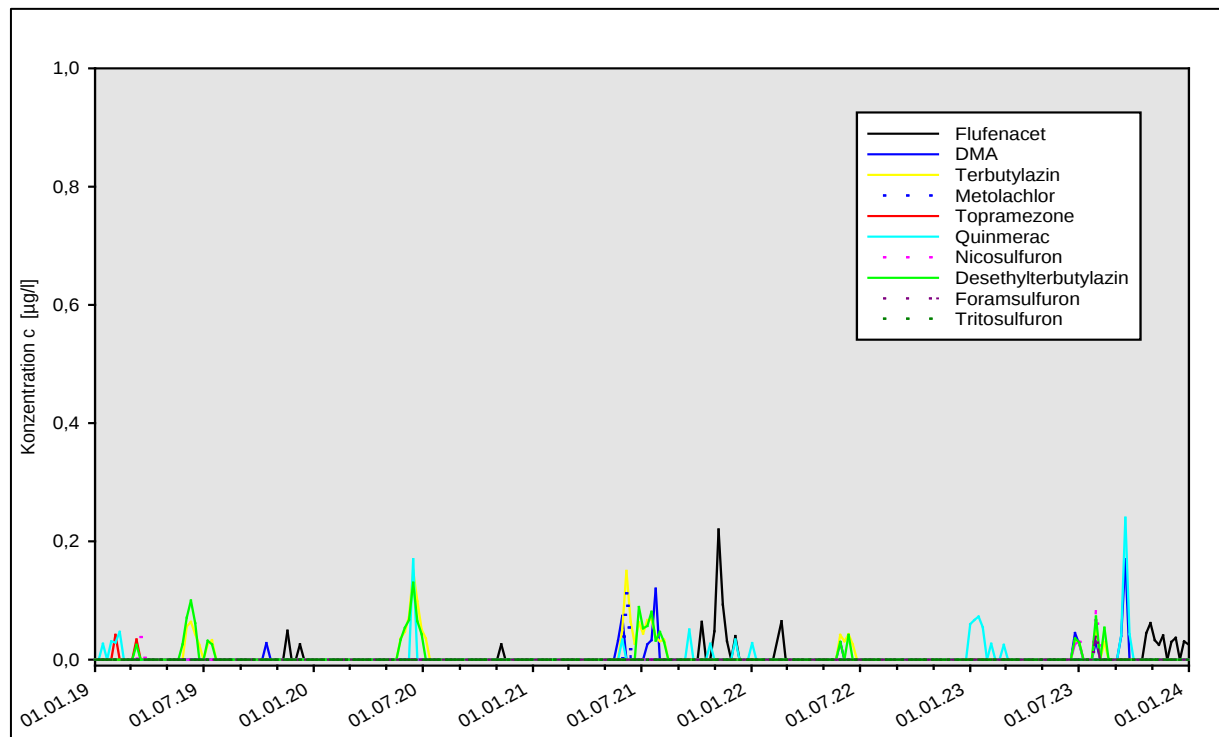
Bild 9: PSM-Befunde in der MP Stever-Senden
