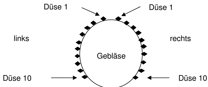
Bild 1 : Düsenanordnung an einer Sprühmaschine
