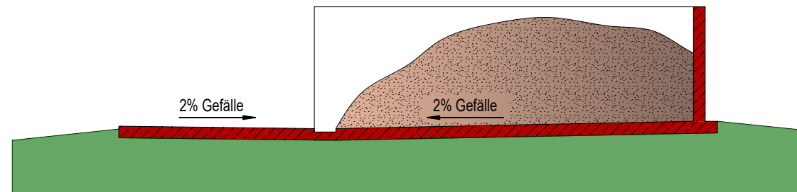
Querschnitt Festmistlager mit Jauchebehälter
