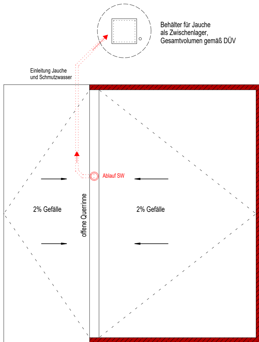
Grundriss Festmistlager mit Jauchebehälter
